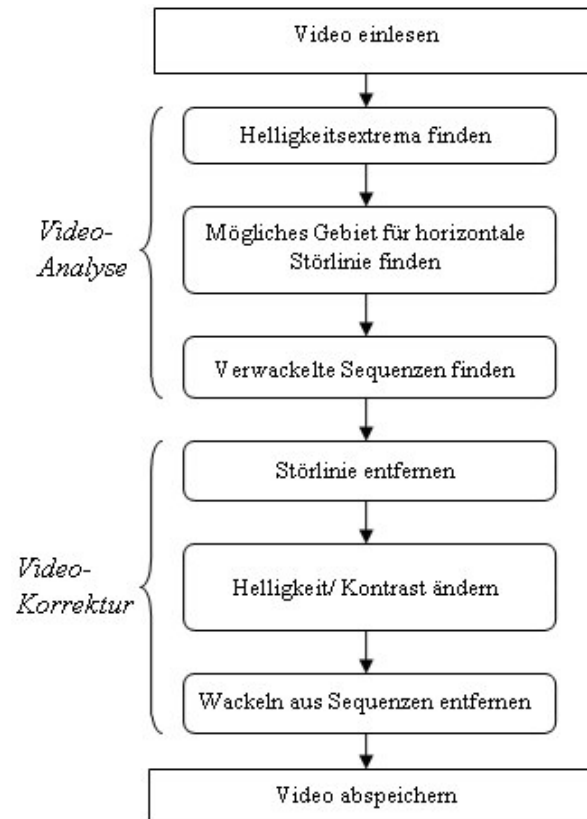
Abbildung 1: Gesamtüberblick über das Programm
