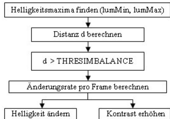
Abbildung 3: Ablauf der Helligkeitskorrektur
