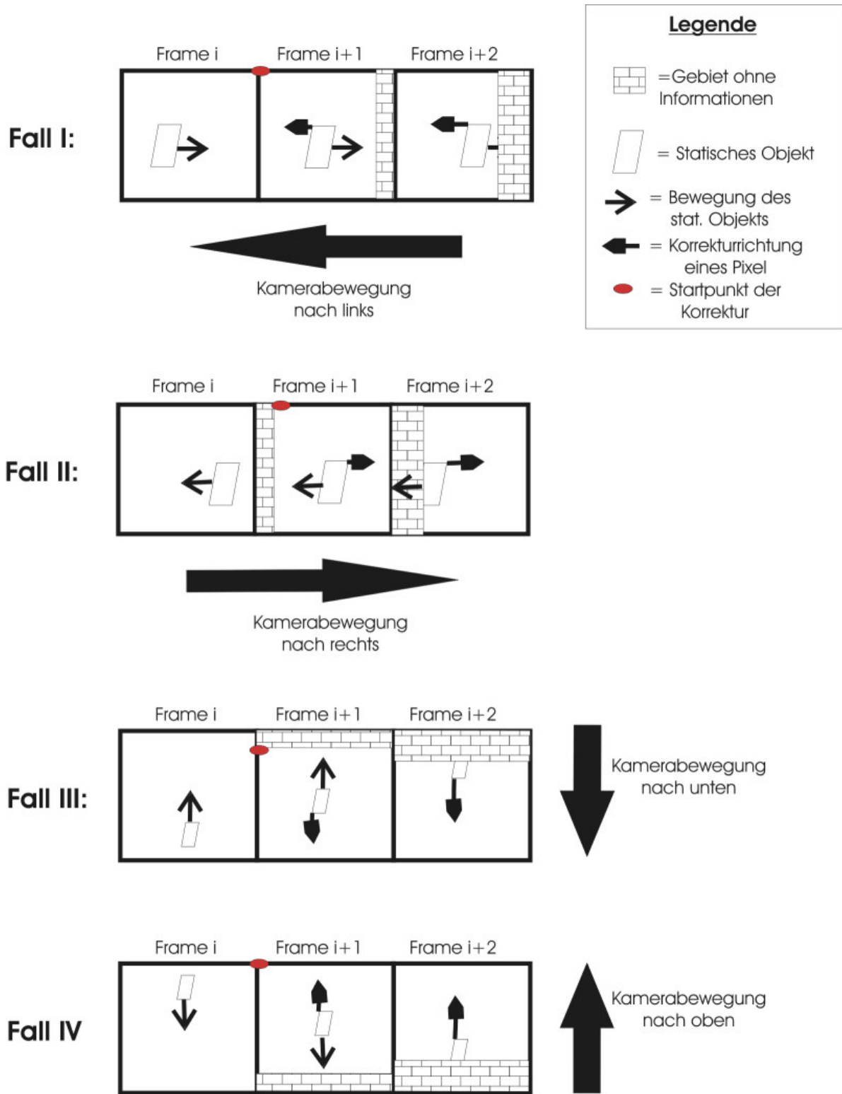
Abbildung 10: Die 4 Fälle der Kamerabewegungen und deren Korrekturen
